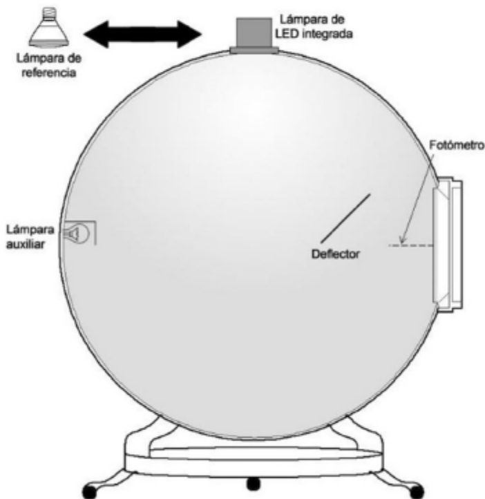
Figura K2 - Configuración de la esfera integradora 2π
